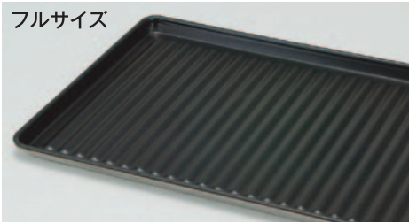
② ノンスティック波型アルミシートパン 68376 フルサイズ ¥18,000 650×450×25mm 板厚1.3mm ●材質:アルミニウム
