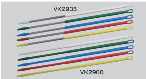
⑧ヴァイカン ハンドル VK2935 重量500g 材質アルミニウム ¥5,000 VK2960 重量415g 材質ポリプロピレン ¥5,900 全長1,300mm 耐熱温度:100℃ カラー:(2935)ホワイト・グリーン・ブルー・レッド・イエロー・オレンジ・パープル・ピンク (2960)ホワイト・グリーン・ブルー・レッド・イエロー
