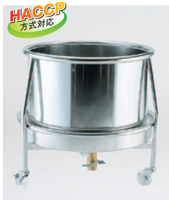
③ざる置台(ドライ用、ステンレスガード付) 392-C φ600(内径550)×600mm ¥110,000 ●材質:ステンレス/パイプφ25mm ※ステンレスガード取り外し可能。 ※キャスターナイロンφ75mm×巾20mm (ストッパー2ヶ付)
