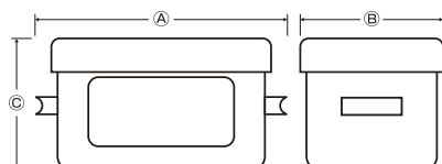
マイルドボックスの最大外形寸法(蓋付)
