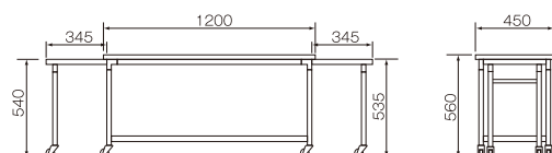
⑤B-2型 両袖式(スチール製折りたたみ) 1200×450×H560mm ¥67,000
