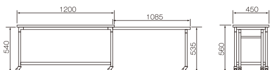
③B-1型 親子式(スチール製折りたたみ) 1200×450×H560mm ¥63,000
