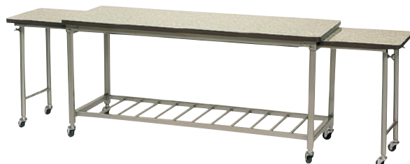
⑤B-2型 両袖式(スチール製折りたたみ) 1200×450×H560mm ¥67,000
