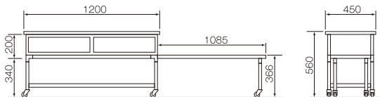
①A-1型 親子式(スチール製折りたたみ) 1200×450×H560mm 抽出2ヶ付き ¥78,000
