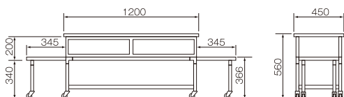
②A-2型 両袖式(スチール製折りたたみ) 1200×450×H560mm 抽出2ヶ付き ¥80,000
