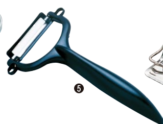
⑤ セラミックピーラー CP-NBK ¥750 サイズ:刃渡り40mm 76×145mm ●材質:刃部/ファインセラミック 柄部/ABS樹脂
