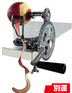
⑳ りんご皮むき機 IS-310 ¥20,000 130×150×高さ200mm 果実直径55~115mm位の梨・りんご専用。
