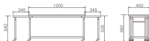
⑤B-2型 両袖式(スチール製折りたたみ) 1200×450×H560mm ¥82,800
